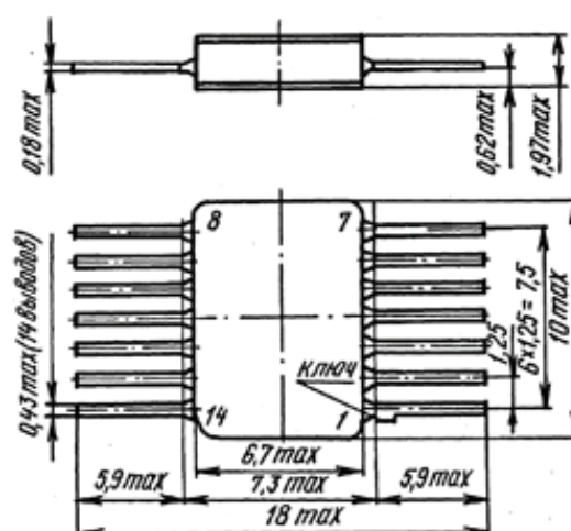
Корпус 401.14-5M
