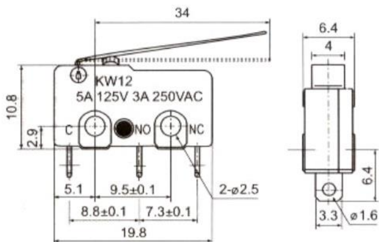
Рис. 2 Схема микропереключателя KW12
