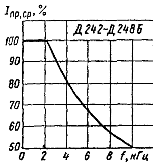
Зависимость среднего прямого тока от частоты
