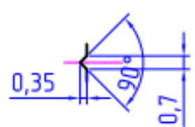
Б (4:1) 3 места
