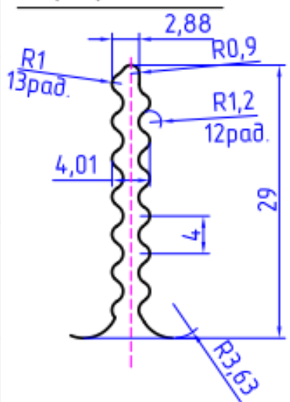
A (2:1) 9 мест
