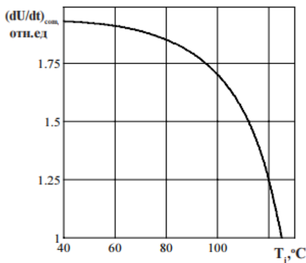
Рисунок 12 - Зависимость критической скорости нарастания коммутационного напряжения (dU_D/dt)_{com} (отн.ед.) от температуры структуры T_j C при I_T = I_{TRMS} , t_f = 10\text{ мс} .
