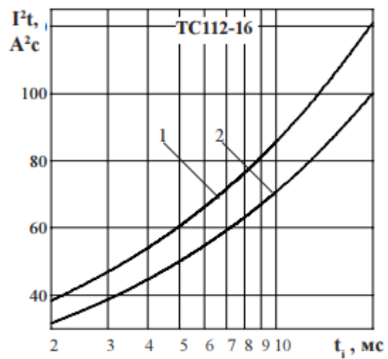
Рисунок 6 - Зависимость защитного показателя \Gamma t от длительности импульса тока t_i при исходной температуре структуры T_j = 25\text{ }^\circ\text{C} (1) и максимальной температуре T_{jm} (2)
