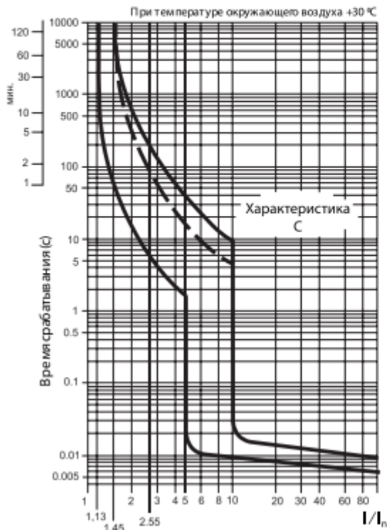
Рисунок 1. Время-токовая характеристика C
