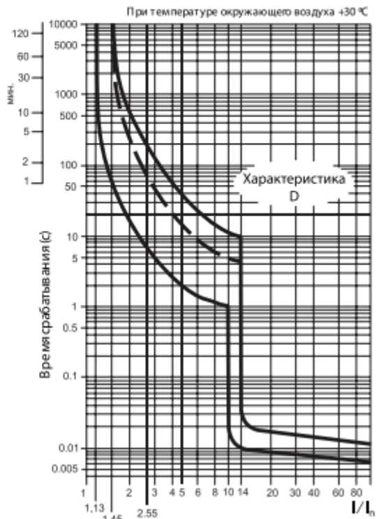
Рисунок 2. Время-токовая характеристика D
