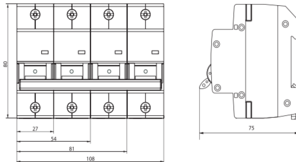
Рисунок 5. Габаритные размеры, мм
