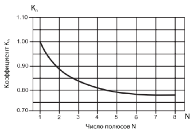
Рисунок 3. Коэффициент, учитывающий количество параллельно размещенных выключателей
