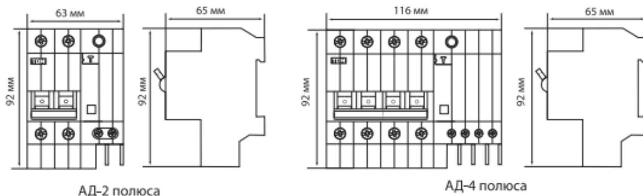
Рисунок 2. Габаритные размеры
