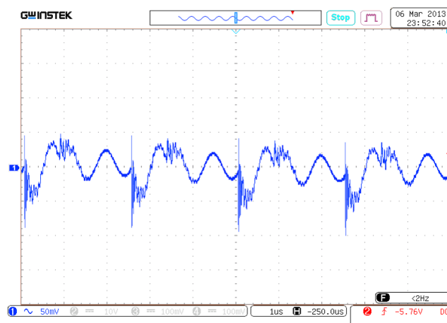
Рис. 31. Пульсации U_{\text{вых.ном}} . Масштаб 50 мВ/дел. Развертка 1 мкс/дел.
