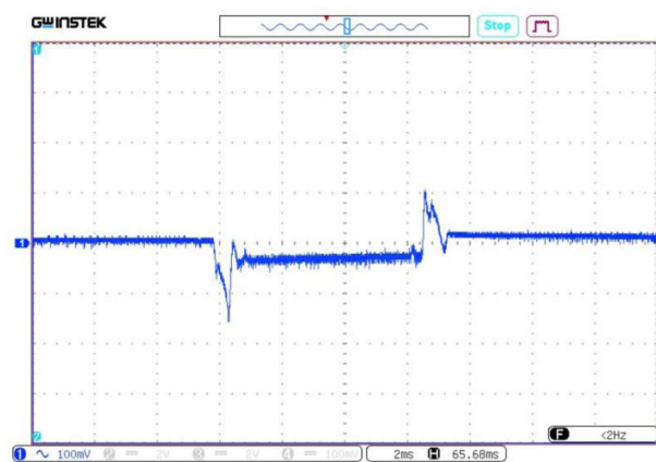
Рис. 29. Осциллограмма переходного отклонения выходного напряжения при скачкообразном изменении выходного тока с 50% до 100% и со 100% до 50%. Масштаб 100 мВ/дел. Развертка 2 мкс/дел.
