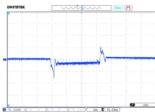
Рис. 25. Осциллограмма переходного отклонения выходного напряжения при скачкообразном изменении выходного тока с 50% до 100% и со 100% до 50%.
