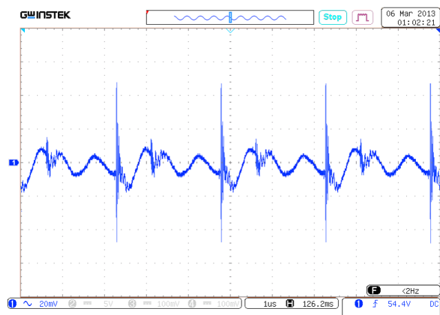
Рис. 27. Осциллограмма пульсаций U_{\text{вых.ном}} . Масштаб 20 мВ/дел. Развертка 1 мкс/дел.
