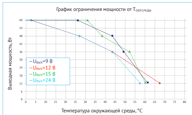
Рис. 23. График ограничения мощности от T_{окр.среды} без применения внешнего радиатора. Для модулей VDRI60W с входной сетью «W», при U_{BX}=48 В .
