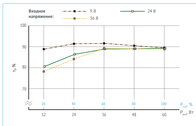
Рис. 14. КПД для VDRI60B15.
