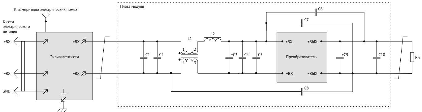
Рис. 4. Схема включения VDRI40, VDRI60 для соответствия стандарту EN 55032 Class B.
