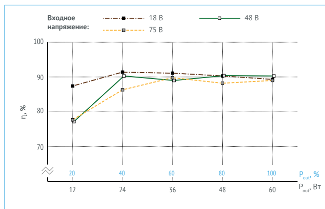
Рис. 18. КПД для VDRI15W09.
