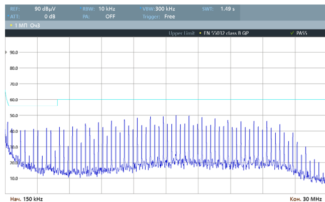
Рис. 45. Спектрограмма работы VDRI60B15 по схеме включения [Рис. 4], измерения произведены в соответствии с EN 55032 Class B (0,15–30 МГц).
