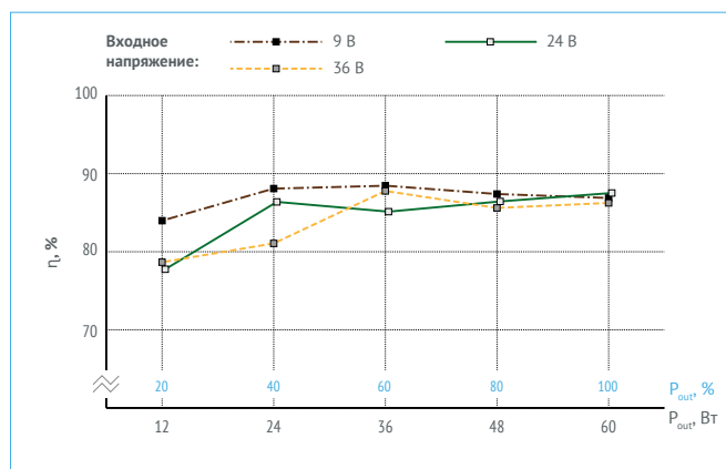
Рис. 16. КПД для VDRI60B48.
