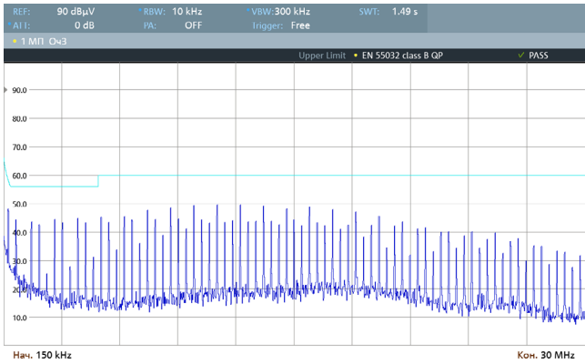
Рис. 47. Спектрограмма работы VDRI60W15 по схеме включения [Рис. 4], измерения произведены в соответствии с EN 55032 Class B (0,15–30 МГц).
