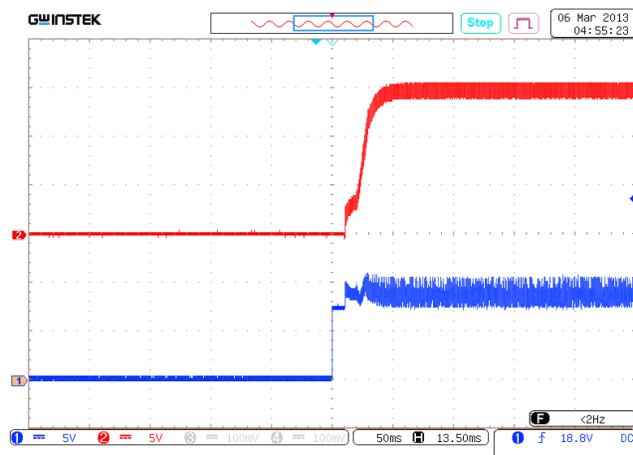
Рис. 24. Установление U_{вых.ном} с момента подачи сигнала ДУ (размыкание выводов «ДУ» и «-ВХ»).
