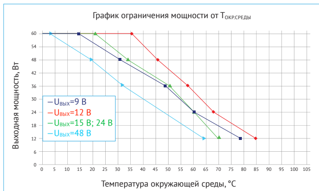
Рис. 22. График ограничения мощности от T_{окр.среды} без применения внешнего радиатора. Для модулей VDRI60B с входной сетью «В», при U_{BX}=24 В .
