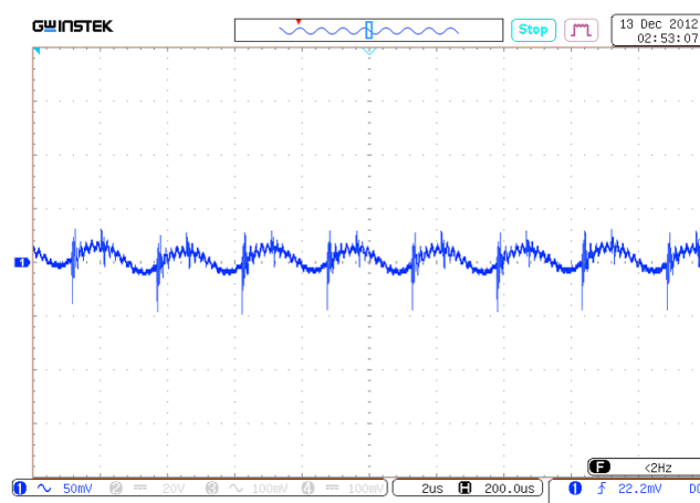
Рис. 35. Пульсации U_{\text{вых.ном}} . Масштаб 10 мВ/дел. Развертка 2 мкс/дел.
