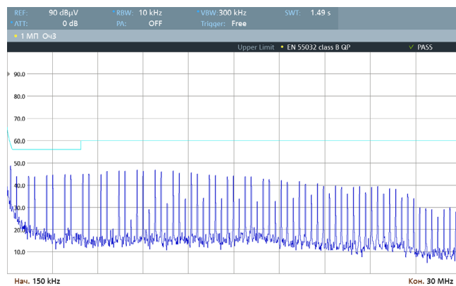
Рис. 43. Спектрограмма работы VDRI40W15 по схеме включения [Рис. 4], измерения произведены в соответствии с EN 55032 Class B (0,15–30 МГц).
