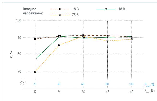
Рис. 20. КПД для VDRI60W15.
