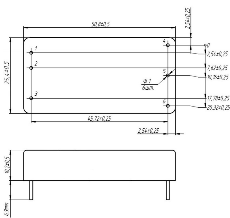
Рис. 48. Исполнение VDRI40, VDRI60.
