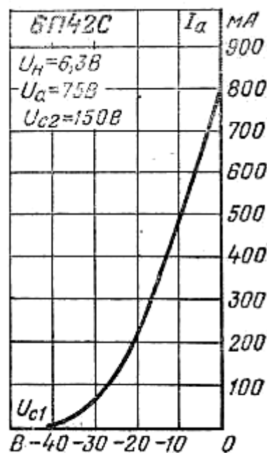
Анодно-сеточная характеристика.
