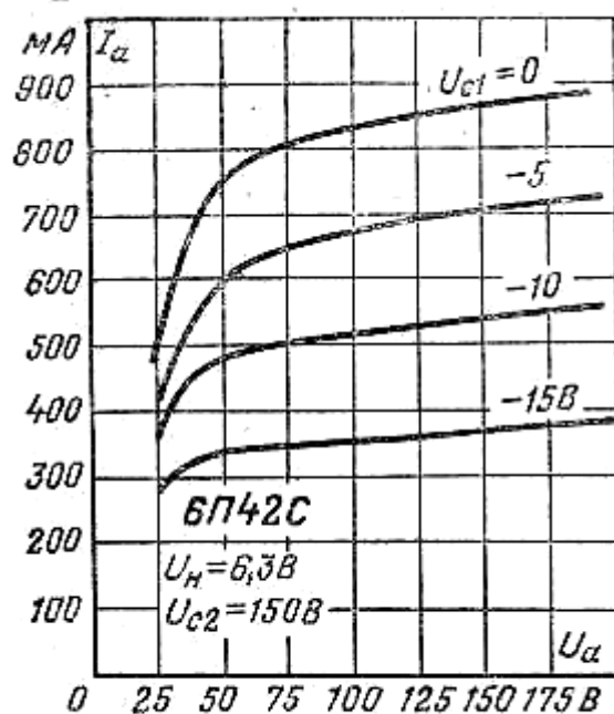
Анодные характеристики.
