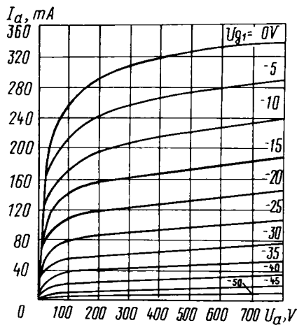
Усредненные анодные характеристики (по сетке второй): U_i = 12,6 \text{ В}; U_{g2} = 250 \text{ В}; U_{g3} = 0 \text{ В} Averaged Anode-Grid 2 Characteristic Curves: U_i = 12.6 \text{ V}; U_{g2} = 250 \text{ V}; U_{g3} = 0
