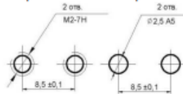
Разметка для крепления
