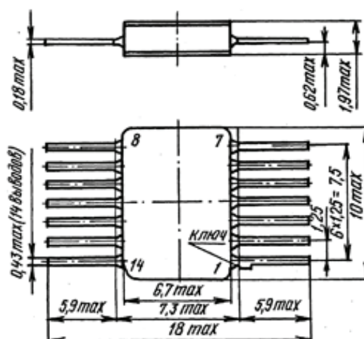
Корпус 401.14-5М
