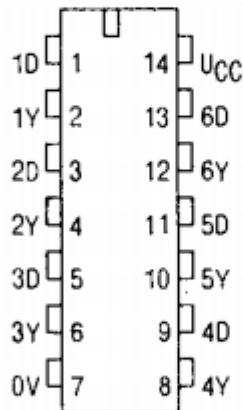
Расположение выводов
