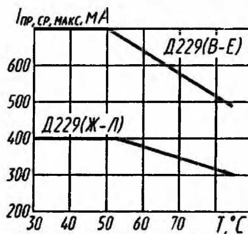
Зависимости допустимого прямого тока от температуры
