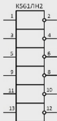
Распиновка К561ЛН2
