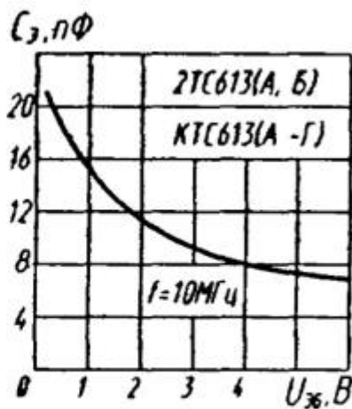
Зависимость емкости эмиттерного перехода от напряжения эмиттер—база
