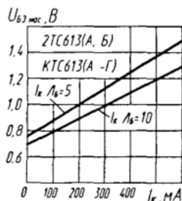
Зависимости напряжения насыщения база—эмиттер от тока коллектора
