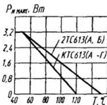
Зависимости допустимой импульсной рассеиваемой мощности от температуры
