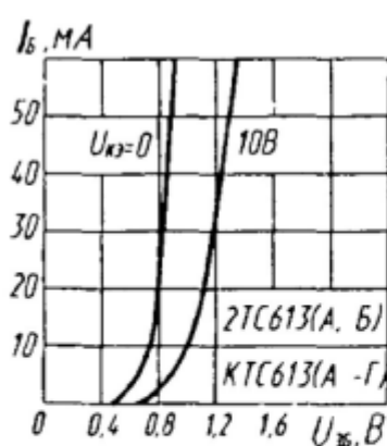
Зависимости тока базы от напряжения база—эмиттер
