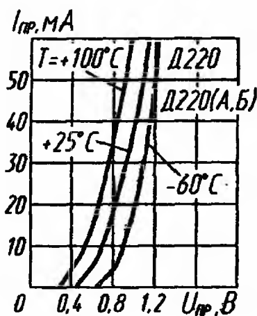
Зависимости прямого тока от прямого напряжения
