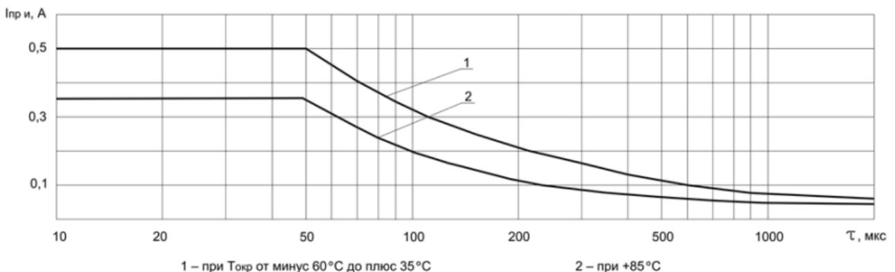
Зависимость максимально допустимого импульсного прямого тока от длительности импульса диодов 3Л118А, АЛ118 при скважности не менее 20
