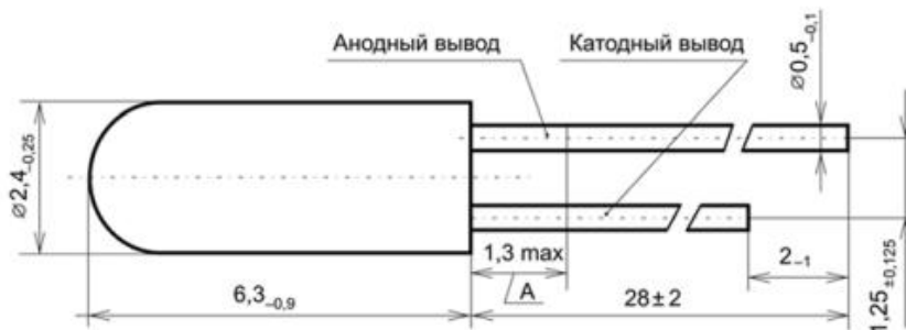
Габаритный чертеж диодов АЛ118 (вариант исполнения ФЫ3.368.006 ГЧ), 3А118
