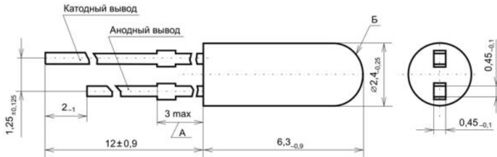
Габаритный чертеж диодов АЛ118 (вариант исполнения ФЫ3.368.006-01ГЧ)
