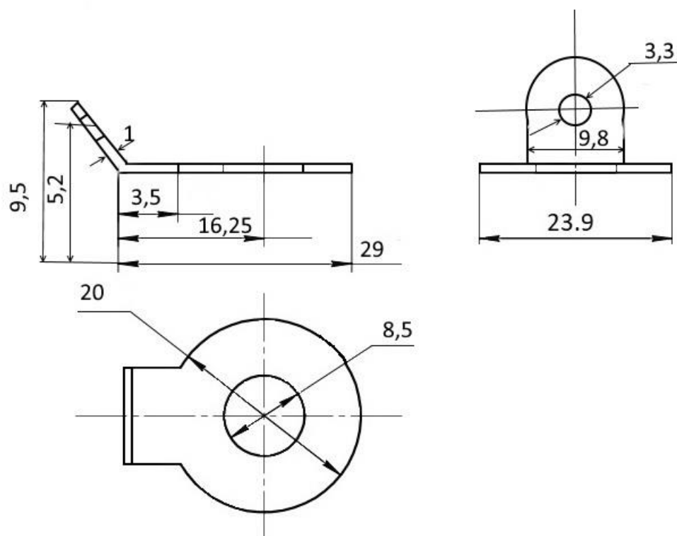
Рис. 2 – Схема токоотвода М6
