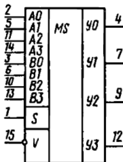
Условное графическое обозначение К555КП16
