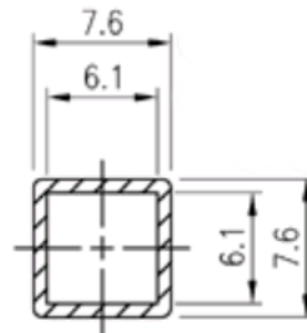
A-A Section
