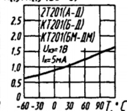
h_{213}/h_{213}(25^\circ\text{С})
