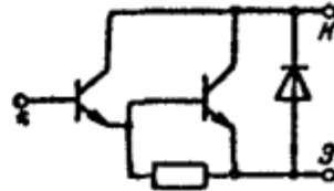
Электрическая схема транзистора КТ972 (А, В)
