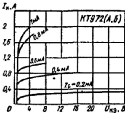
Выходные характеристики
