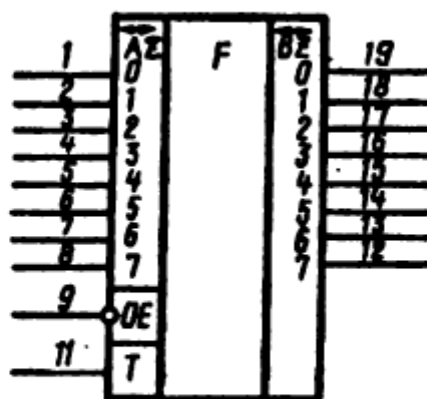
Условное графическое обозначение КМ580ВА86, КР580ВА86
