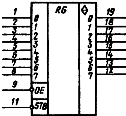
Условное графическое обозначение КР580ИР82
