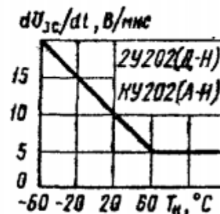
Зависимость скорости нарастания напряжения в закрытом состоянии от температуры корпуса
