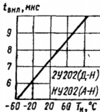
Зависимость времени включения от температуры корпуса
