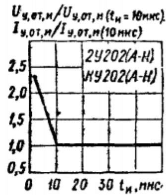
Зависимость отпирающего импульсного тока и напряжения управления от длительности импульса
