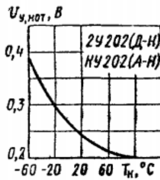
Зависимость неотпирающего постоянного напряжения управления от температуры корпуса
