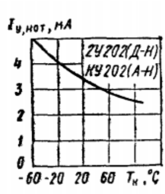
Зависимость неотпирающего постоянного тока управления от температуры корпуса
