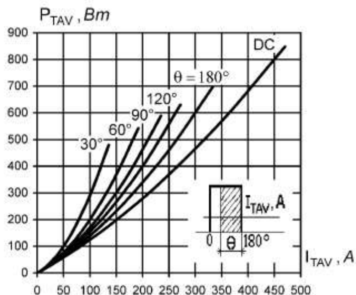
Рис. 6. Мощность потерь в открытом состоянии (прямоугольный импульс)
