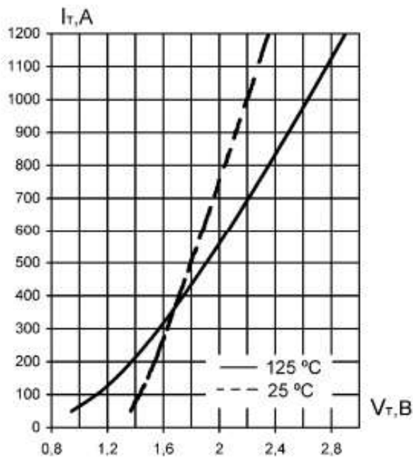
Рис. 1. Предельные вольт-амперные характеристики в открытом состоянии
