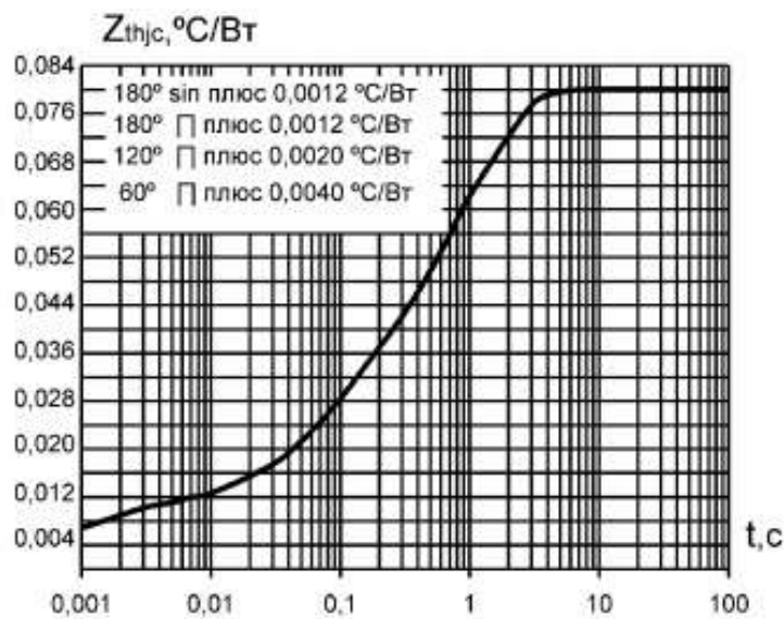
Рис. 2. Переходное тепловое сопротивление переход-корпус ( постоянный ток )
