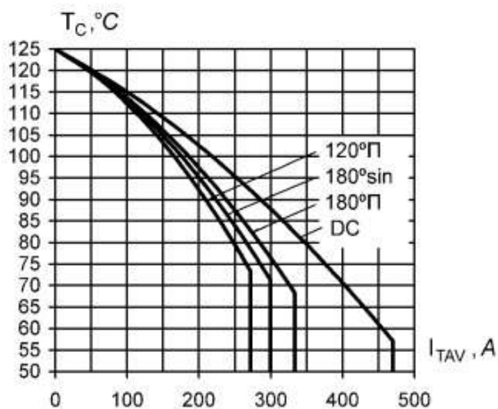
Рис. 7. Максимально допустимая температура корпуса при различных углах управления и различных формах тока
