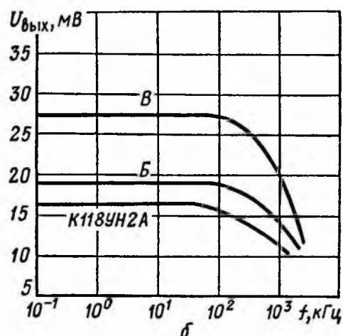
Амплитудные (а) и амплитудно-частотные (б) характеристики ИМС К118УН2
