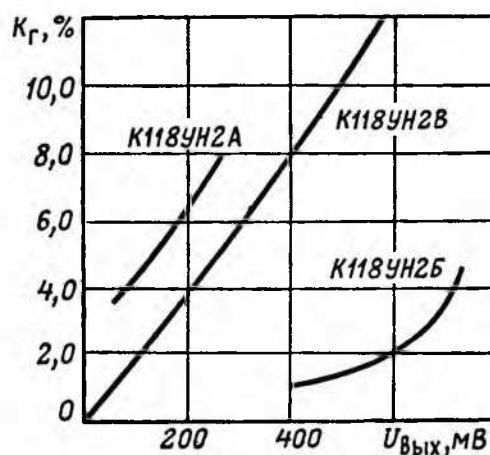
Зависимость коэффициента гармоник ИМС К118УН2 от выходного напряжения
