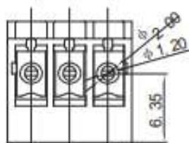
A 向视图
