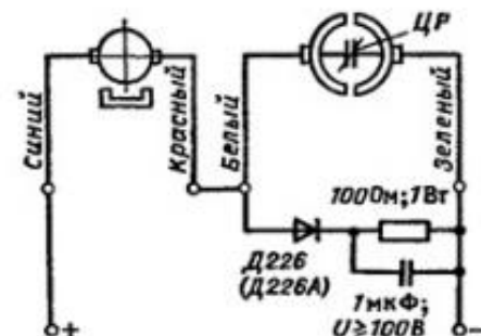
Схема включения двигателей ДПМ-25-НЗ-03:
