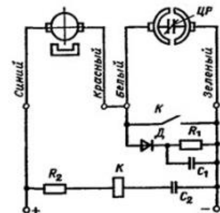
Схема включения двигателей ДПМ-25-НЗ-03:
