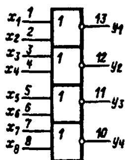
Условное графическое обозначение К115ЛЕ1
