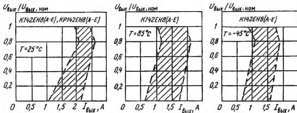
Выходные характеристики ИМС К142ЕН8
