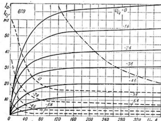
Рис. 404. Усредненные характеристики зависимости тока анода и тока второй сетки от напряжения на аноде при напряжении на второй сетке 150 в: — ток в цепи анода; — ток в цепи второй сетки; — наибольшая мощность, рассеиваемая на аноде.
