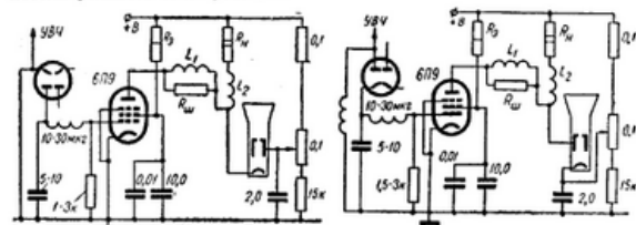
Рис. 399. Схема применения лампы 6П9 для работы в режимах I—III. Рис. 400. Схема применения лампы 6П9 для работы в режимах IV и V.
