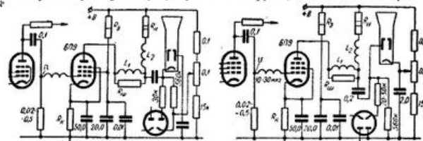
Рис. 401. Схема применения лампы 6П9 для работы в режимах VI и VII. Рис. 402. Схема применения лампы 6П9 для работы в режиме VIII.
