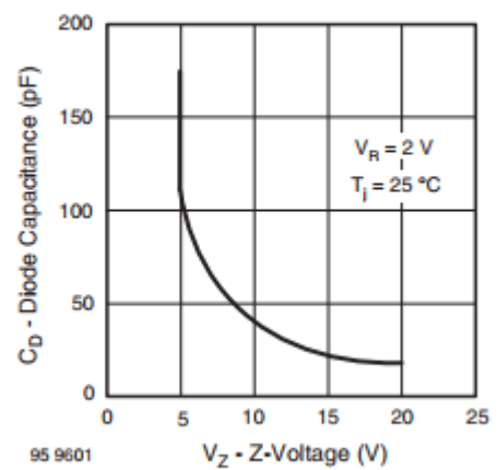
Fig. 5 - Diode Capacitance vs. Z-Voltage
