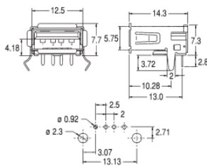
USBA-1J (USB, тип A)
