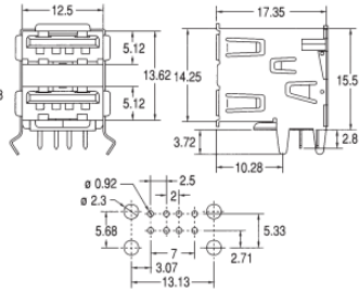
USBA-2J (USB, тип A, двойной)
