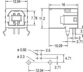
USBB-1J (USB, тип B)
