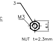
NUT t=2.3mm
