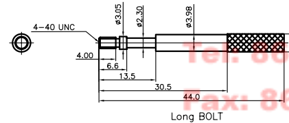
Long BOLT
