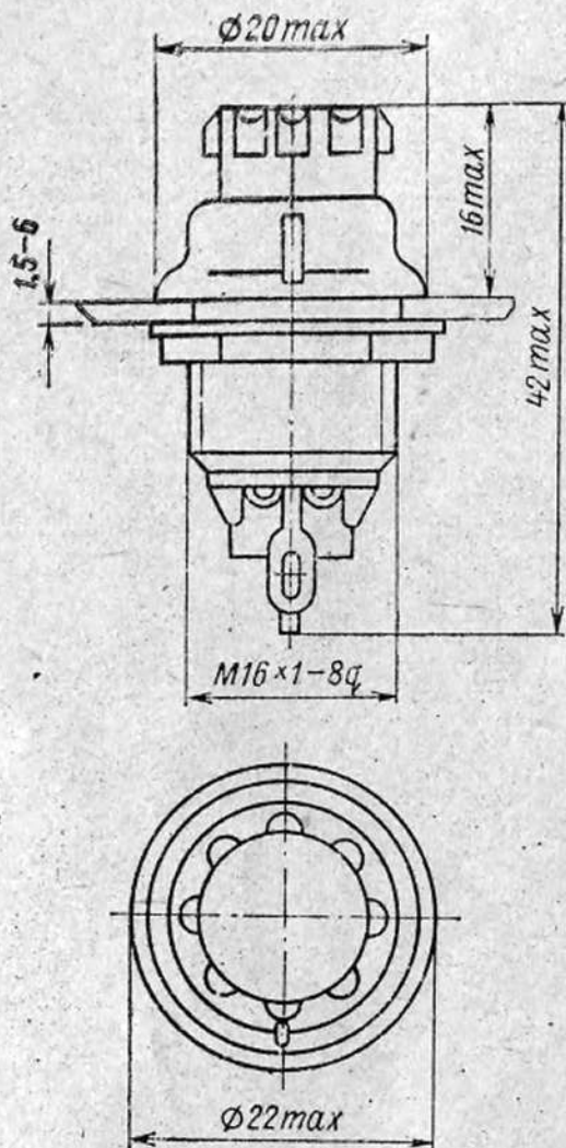
ДП-1Ц
