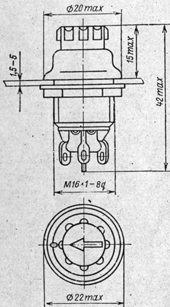
ДП-3
