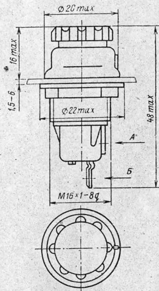
ДП-1ЦМ
