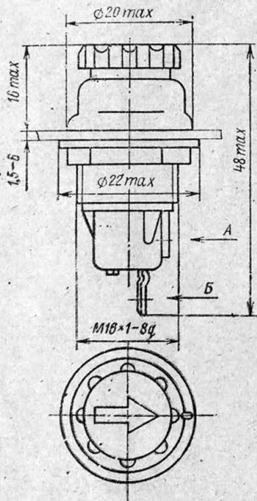
ДП-3М
