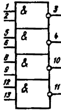
Условное графическое обозначение К561ЛА7, ЭКФ561ЛА7
