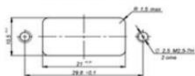
Разметка для крепления РСС 485
