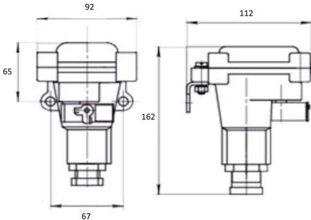
Кнопочный взрывозащищенный пост управления КУ 91 характеристики КУ-91
