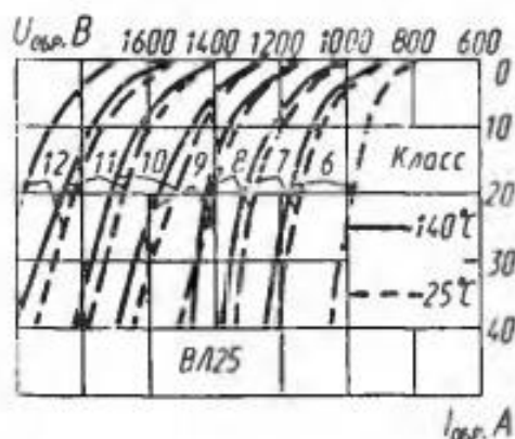
Зависимости обратного напряжения от тока
