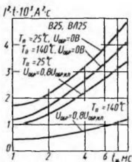
Зависимости защитного показателя от длительности импульса тока
