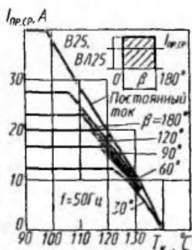
Зависимости допустимого прямого тока от температуры корпуса
