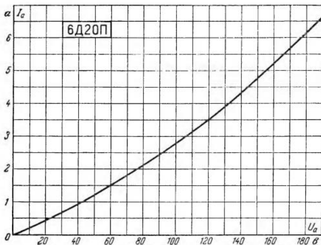
Анодная характеристика лампы 6Д20П.
