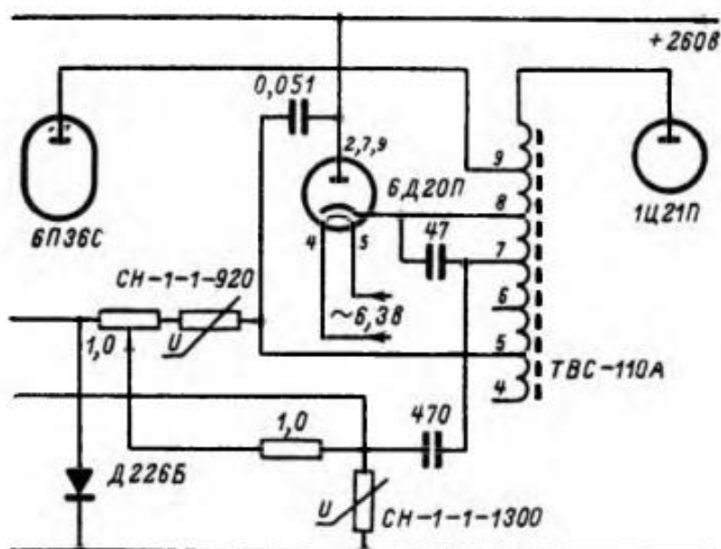
Демпферный диод 6Д20П в выходном каскаде строчной развертки телевизоров УНТ-47 и УНТ-59.
