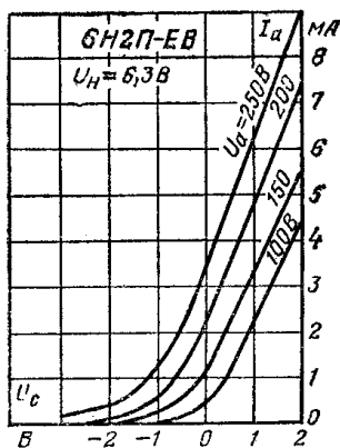
Анодно-сеточные характеристики.
