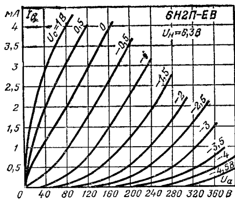
Анодные характеристики.
