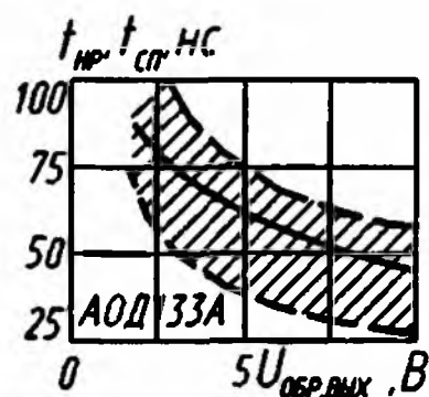
Зона возможных положений зависимости времени нарастания и спада от обратного выходного напряжения
