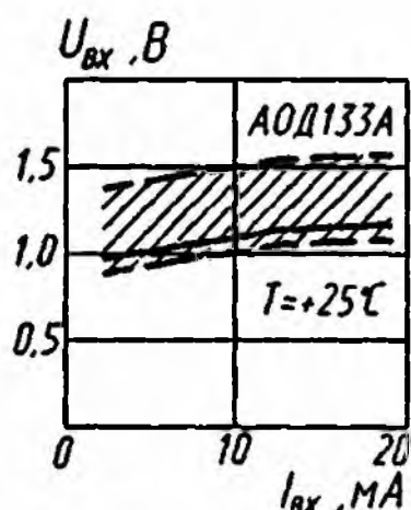
Зона возможных положений зависимости входного напряжения от входного тока
