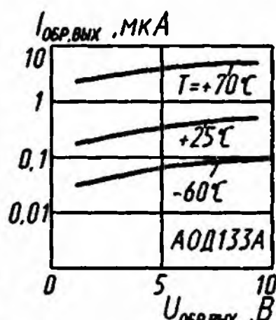
Зависимости обратного выходного тока от обратного выходного напряжения
