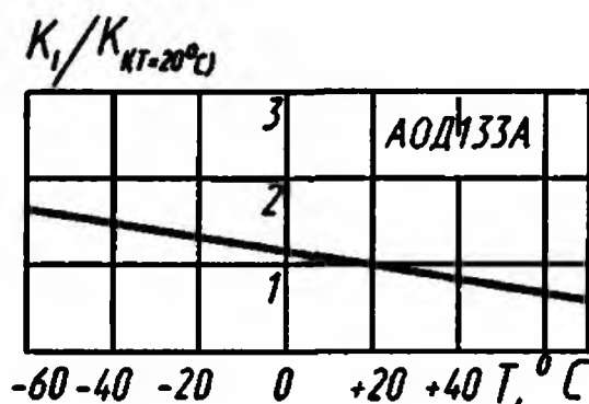
Зависимость относительного коэффициента передачи по току от температуры
