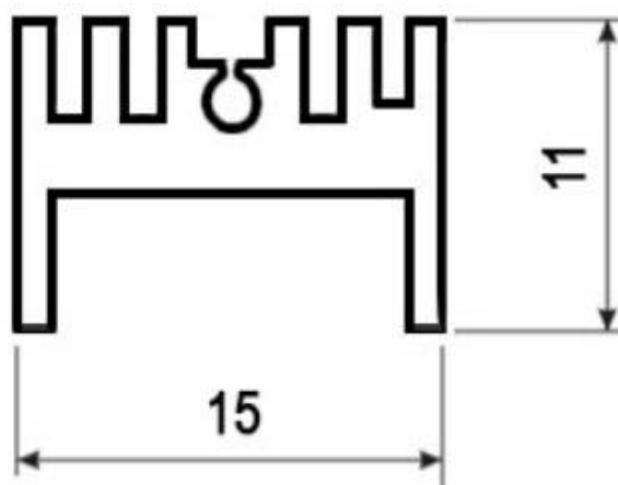
Рис. 2 Схема радиатора BLA002-50 50x15x11mm
