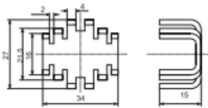
301 27x34x15 mm
