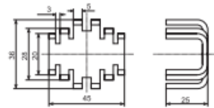
302 36x45x25 mm
