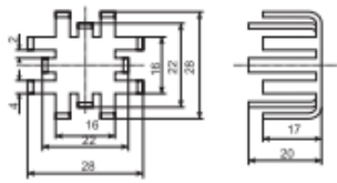
101 28x28x20 mm
