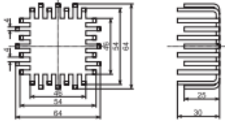
104 64x64x30 mm
