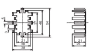
201 38x54x25 mm
