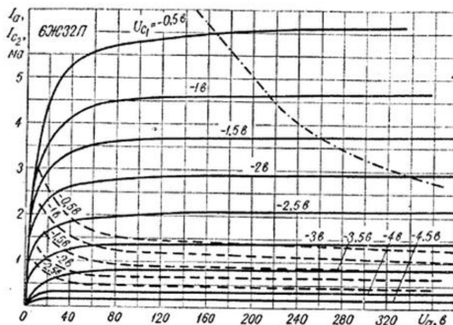
Рис. 266. Усредненные характеристики зависимости тока анода и тока второй сетки от напряжения на аноде при напряжении на второй сетке 140 в: — ток в цепи анода; — — ток в цепи второй сетки; — — — наибольшая мощность, рассеиваемая на аноде.
