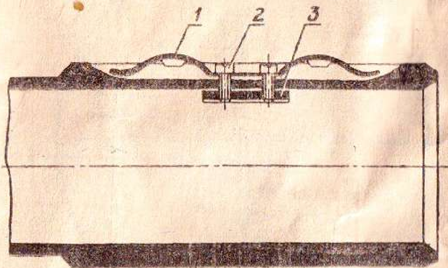
Рис. 5. Замена пружины 1 — пружина; 2 — винт; 3 — планка.
