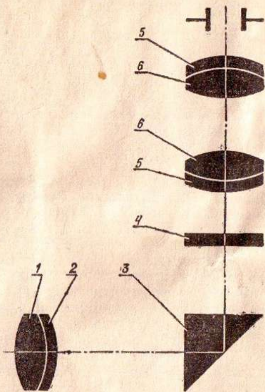
Рис. 1. Оптическая принципиальная схема: 1 — 2 линзы; 3 — призма; 4 — сетка; 5 — 6 линзы
