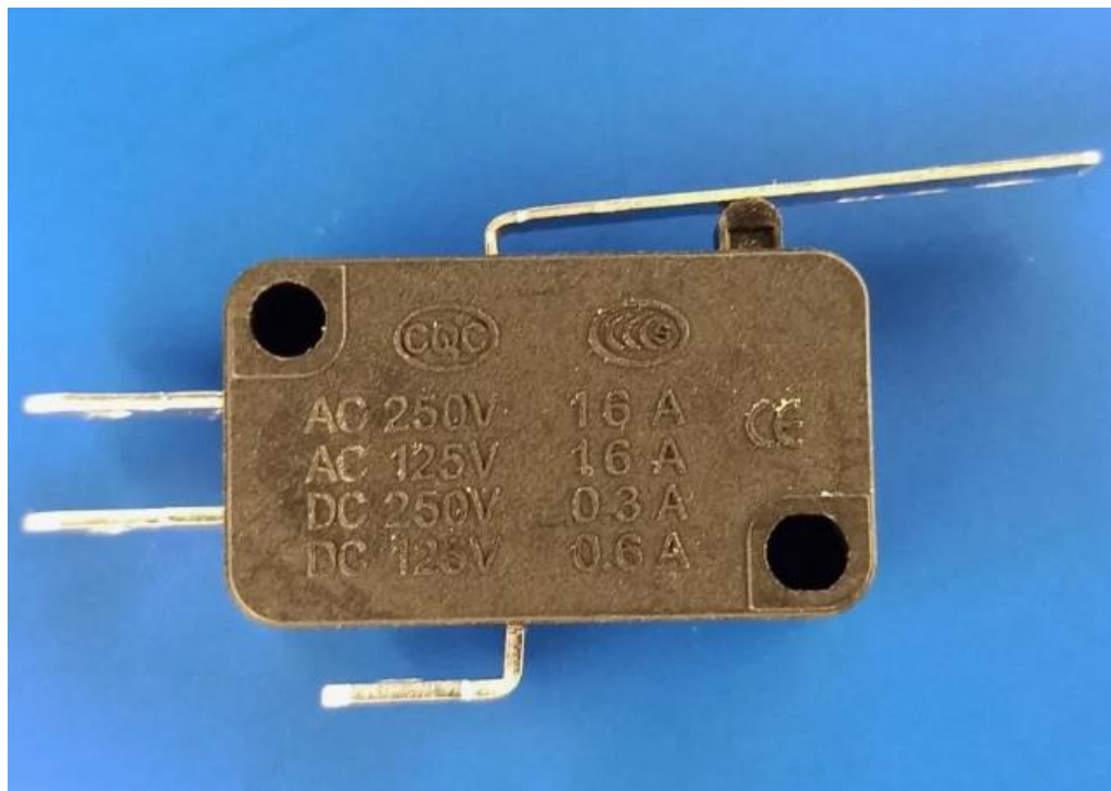
Рис. 1 Микропереключатель KW1-103-1
