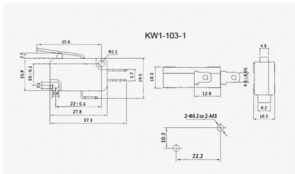
Рис. 2 Схема микропереключателя KW1-103-1
