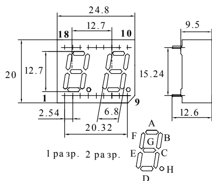
Рис.1 КИПЦ29-2/8 Fig. 1
